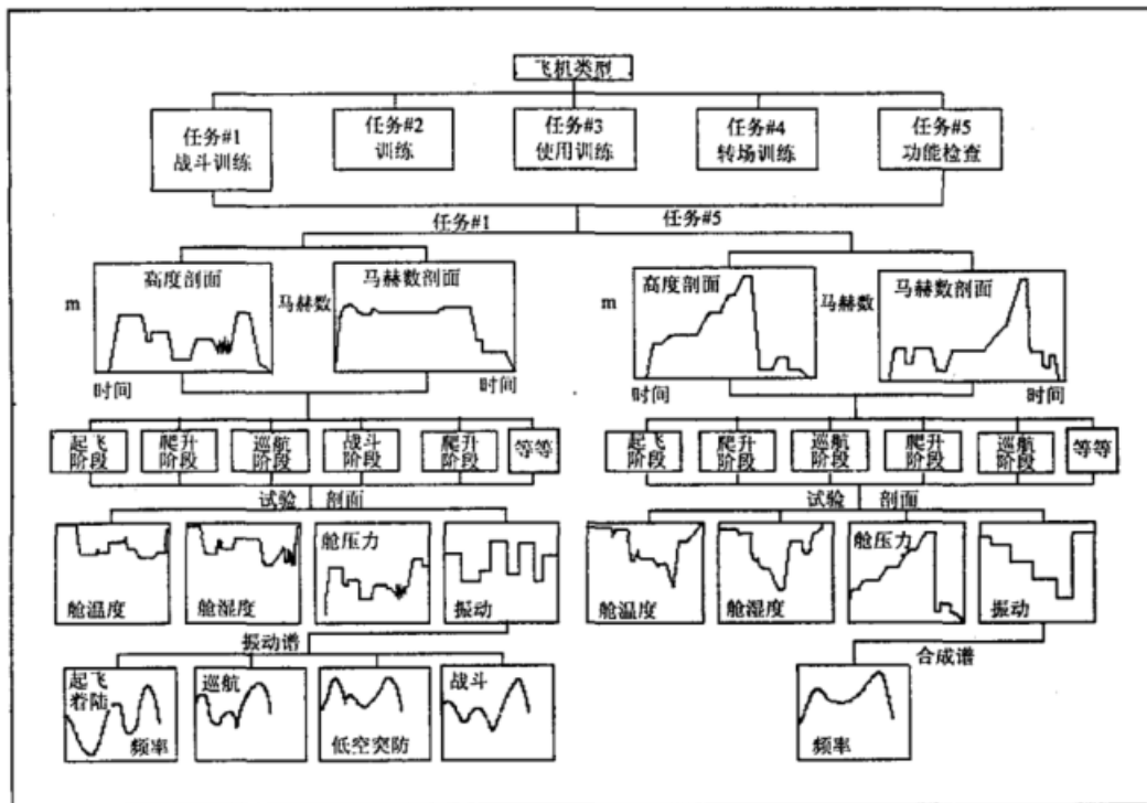
图 1 试验剖面生成流程图
