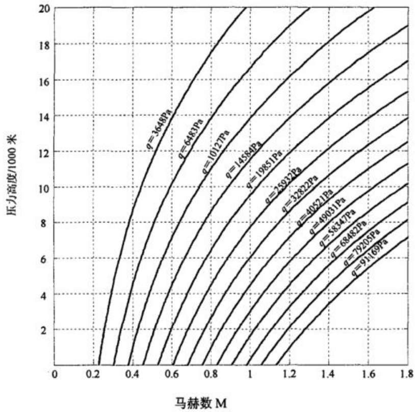
图 4 动压 ( q ) 是马赫数和高度的函数
