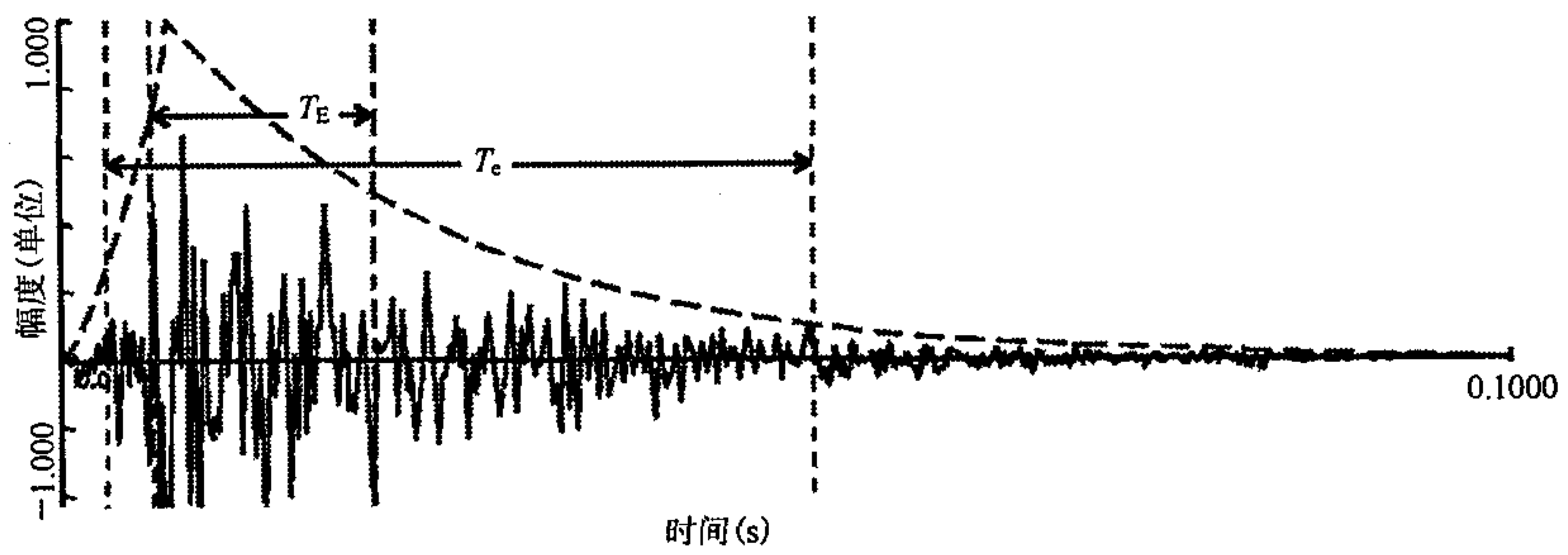
图 C.1 具有包络线的典型冲击时间历程及其 T_E 和 T_e
